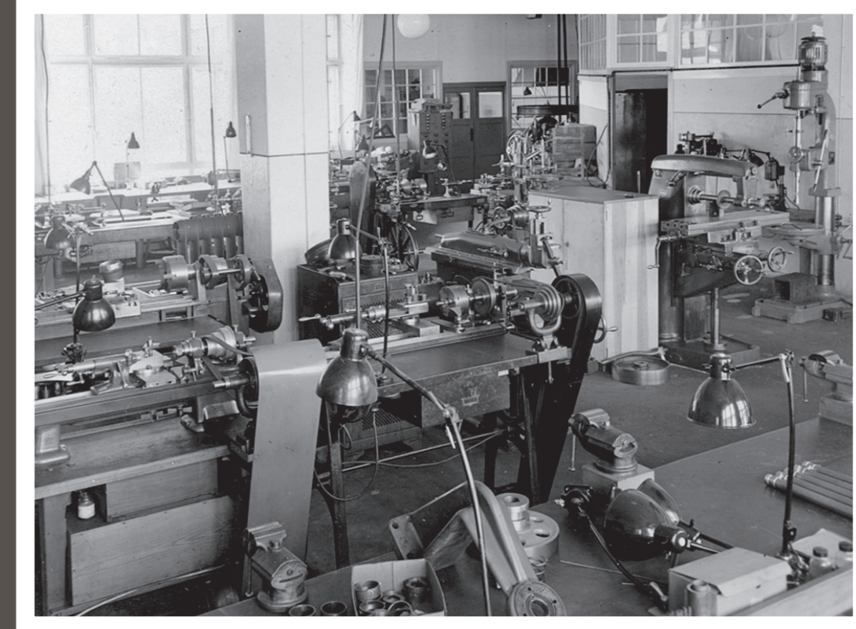
Maschinensaal Berlin Michaelkirchstraße 15 Mechanical turnery Berlin Michaelkirchstraße 15
